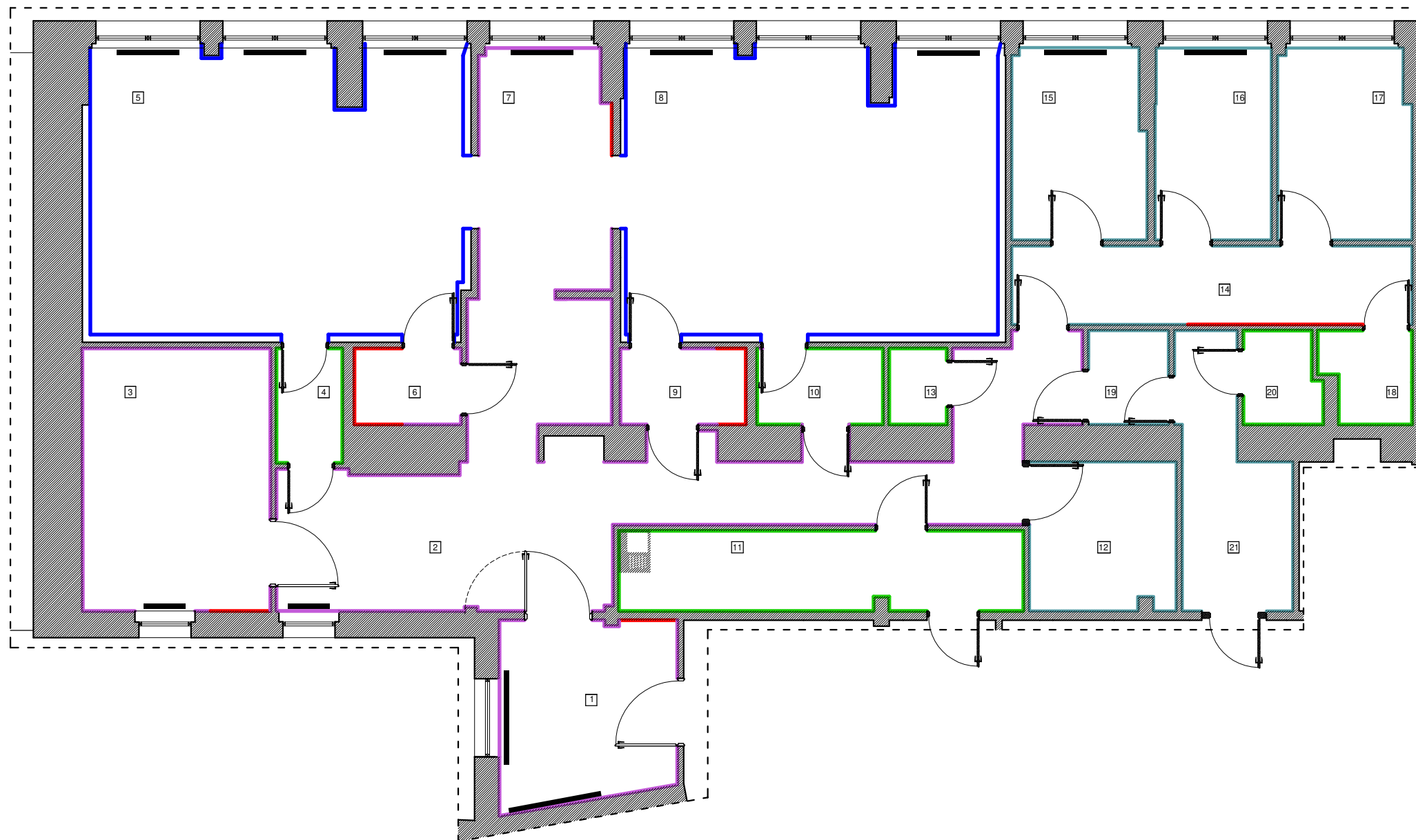
ARANŻACJA WNĘTRZ RYS. NR 2 WYKOŃCZENIA ŚCIAN RZUT BLOKU OPERACYJNEGO
