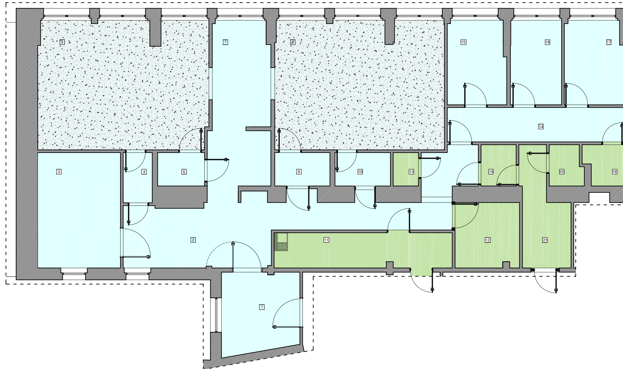
ARANŻACJA WNĘTRZ RYS. NR 4 WYKOŃCZENIA PODŁÓG RZUT BLOKU OPERACYJNEGO
